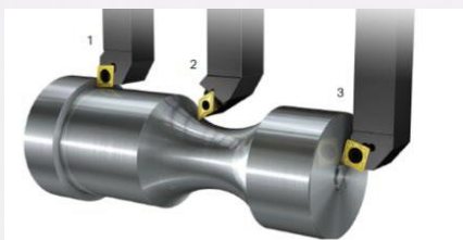
Наружное точение 1. Продольное точение 2. Профильное точение 3. Подрезка торца
