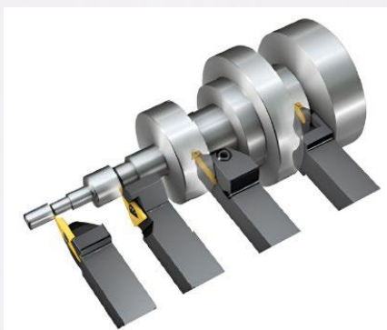
Наружная отрезка и обработка канавок 1. Неглубокая отрезка 2. Средняя отрезка 3. Глубокая отрезка
